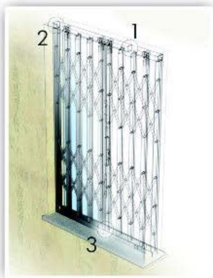
Sistema di appoggio della guida superiore sul montante laterale
