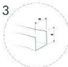
3 profilo a U guida inferiore sez. 50x30 mm (h)
